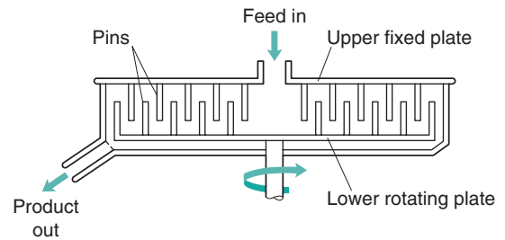
Fig. 10.15 • Pin mill.
