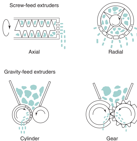
Fig. 28.8 • Production extruders.
