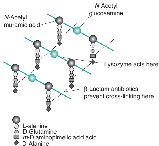
Fig. 13.3 • Peptidoglycan.
