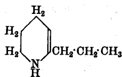
γ-coniceine
