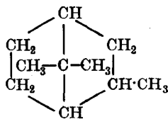
isobornylene
