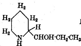
conhydrine
