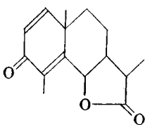
santonin
