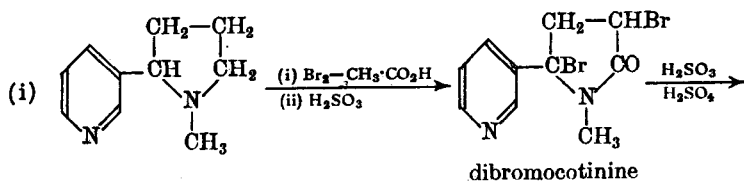
nicotine
