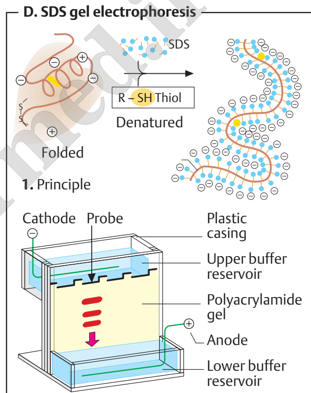
2. Apparatus
