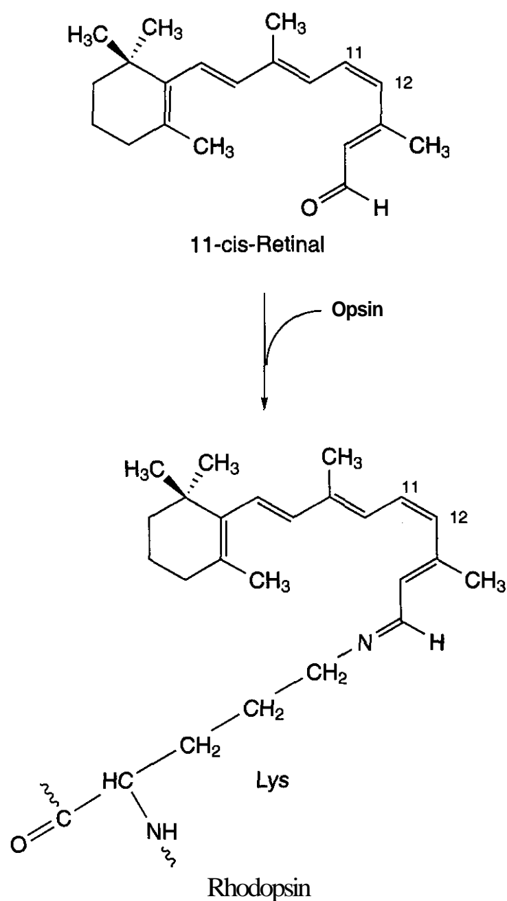
Figure 8.5. Rhodopsin.
