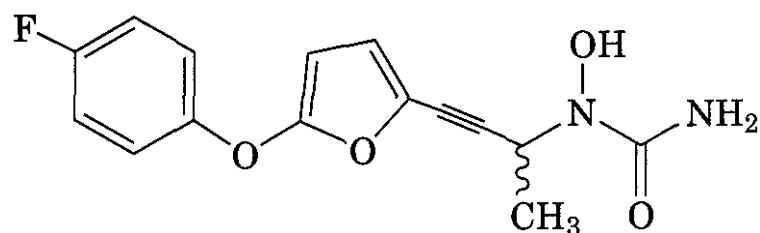
(9) (±) A-78773 R(+) A-79175 S(-) A-79176
