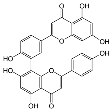
Amentoflavone
